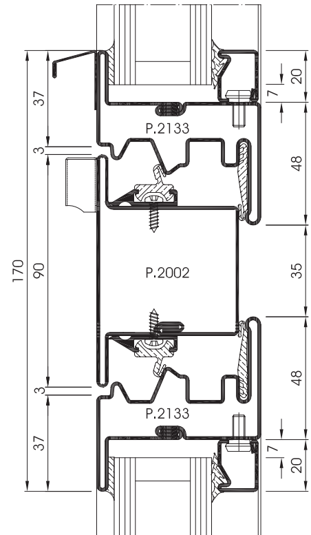
SEZIONE / Section / Schnitt 7
