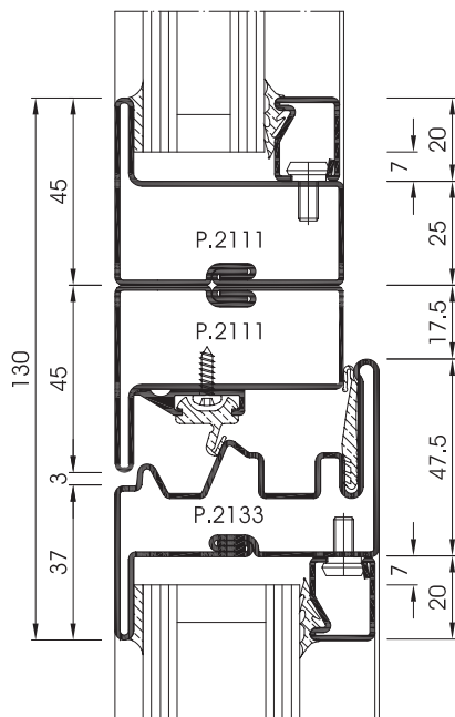
SEZIONE / Section / Schnitt 6
