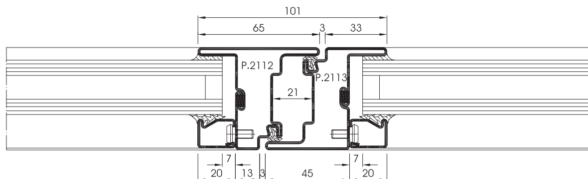
SEZIONE / Section / Schnitt 4
