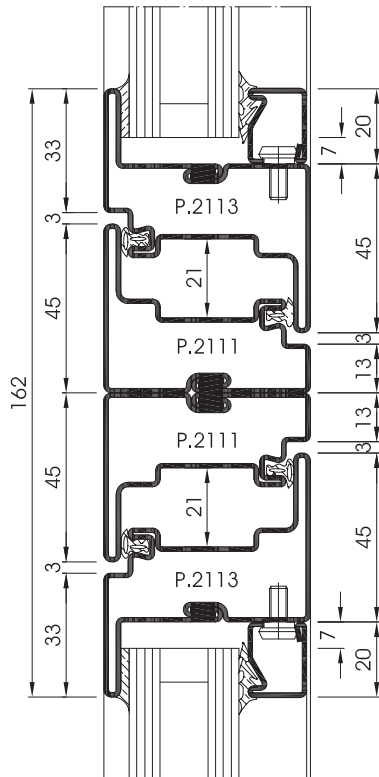
SEZIONE / Section / Schnitt 6
