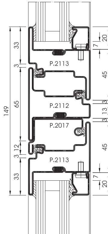
SEZIONE / Section / Schnitt 7
