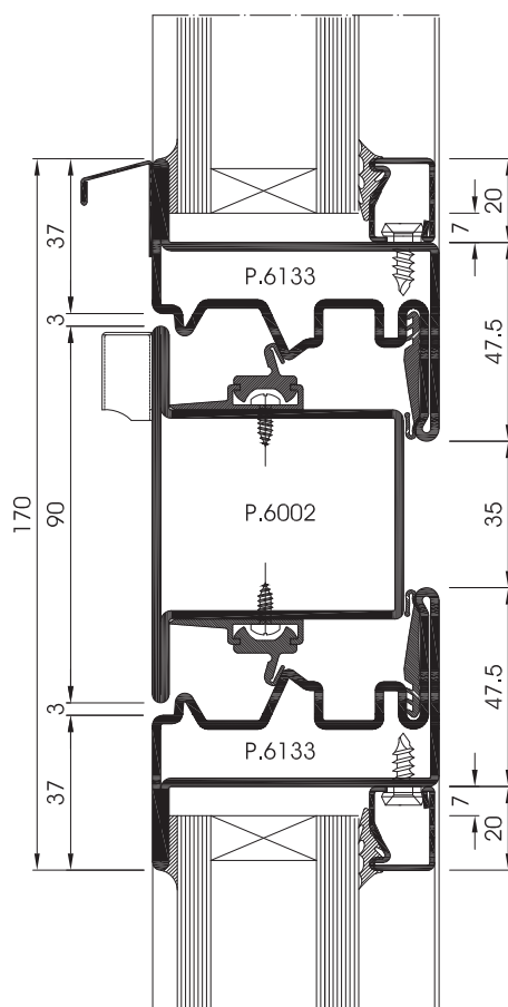
SEZIONE / Section / Schnitt 7
