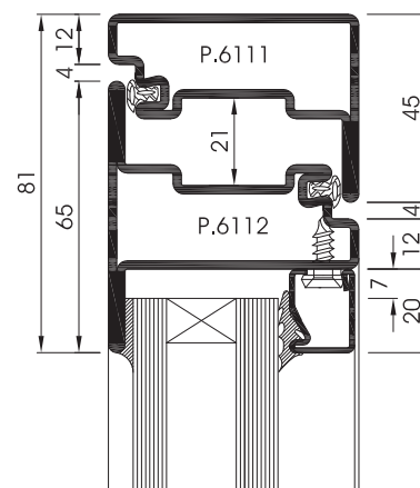
SEZIONE / Section / Schnitt 6a
