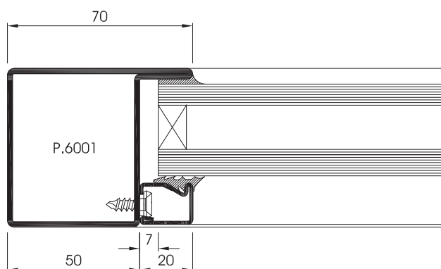
SEZIONE / Section / Schnitt 1
