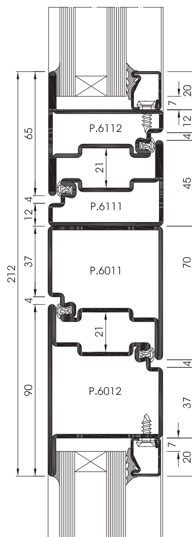
SEZIONE / Section / Schnitt 6a
