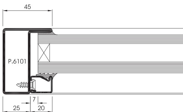
SEZIONE / Section / Schnitt 2
